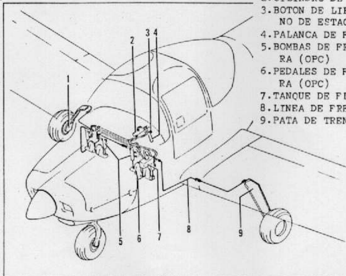
SISTEMA DE FRENOS
